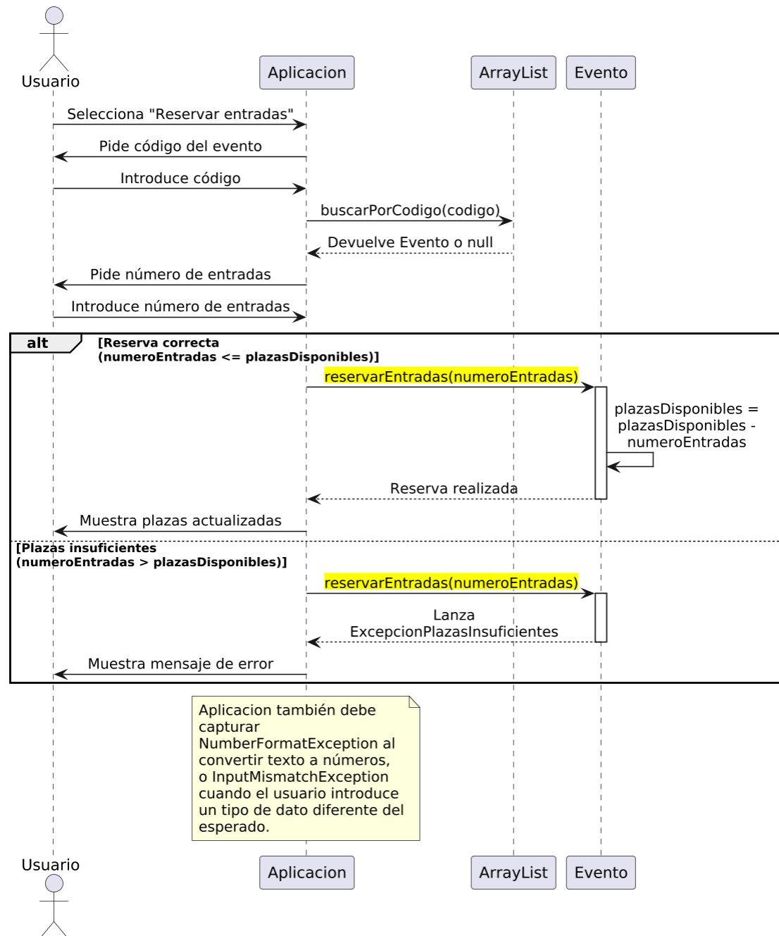
Modalidad D - Diagrama de secuencia de reservarEntradas
